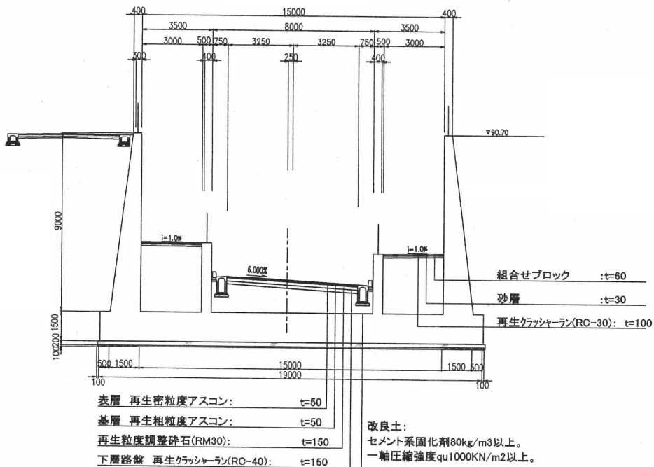
駅北余部線・U型擁壁部 (W=14.5~15.0m)
