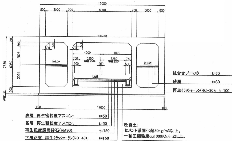
駅北余部線・U型擁壁部 (W=14.5~15.0m)
