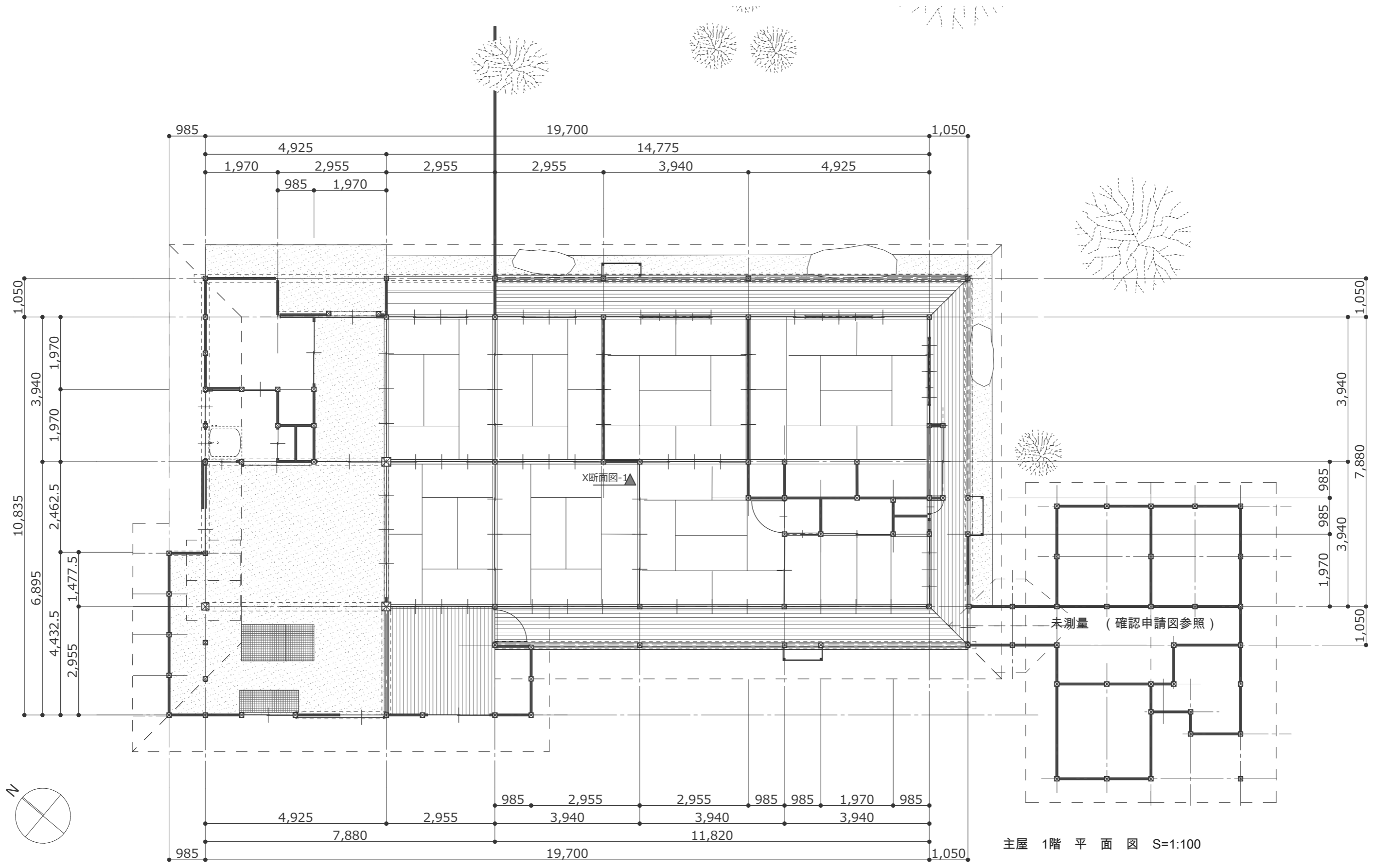
1F 平面図
