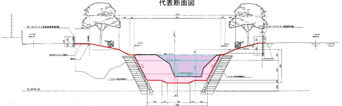
代表断面図
