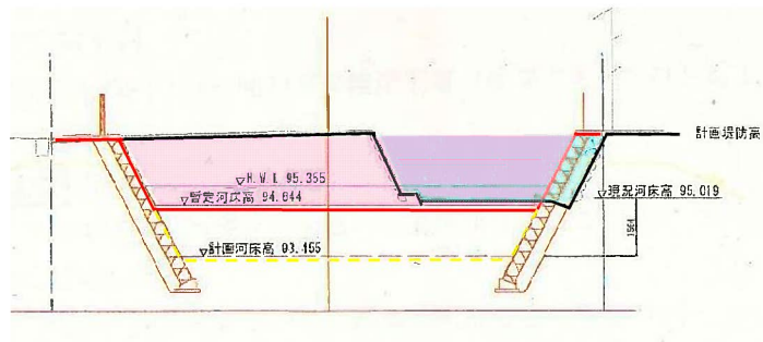
代表断面図
