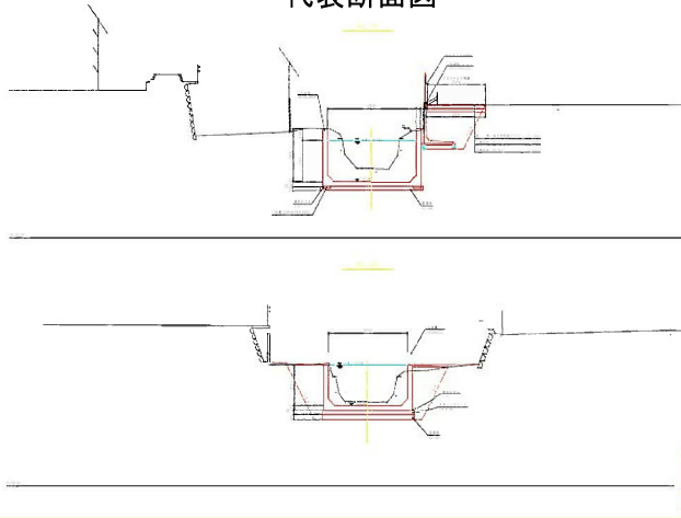
代表断面図
