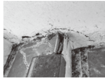
【陸橋のさび】
