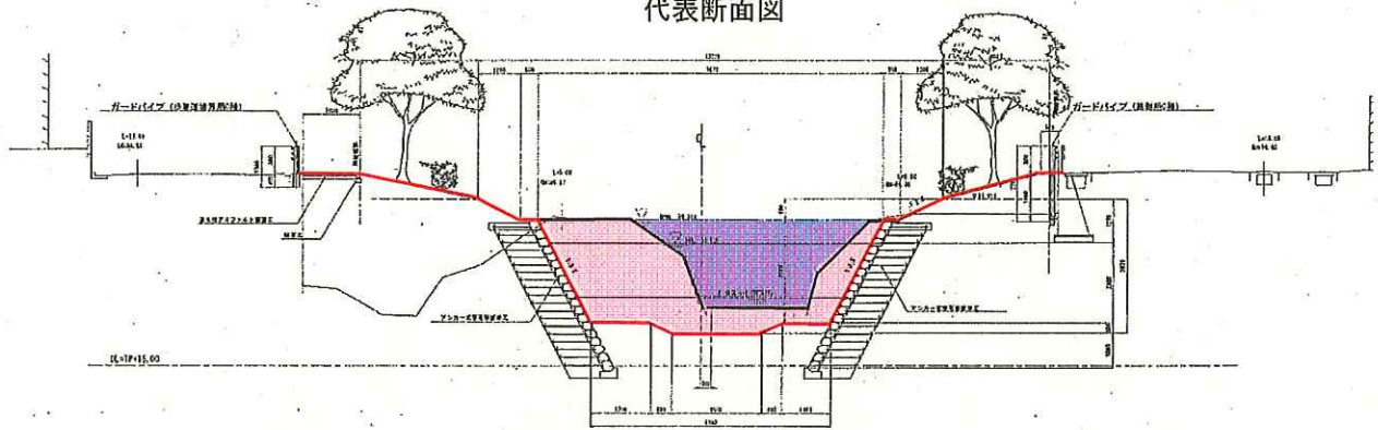
代表断面図
