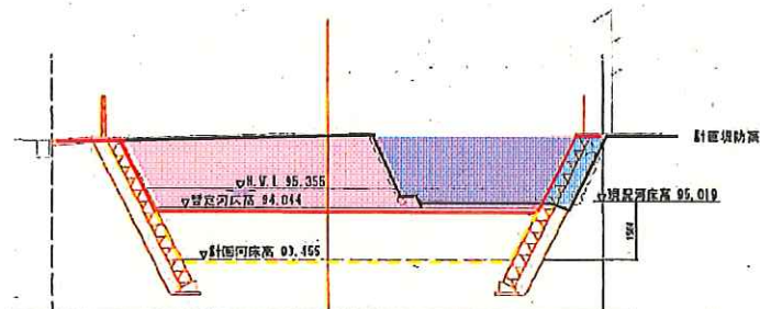
代表断面図
