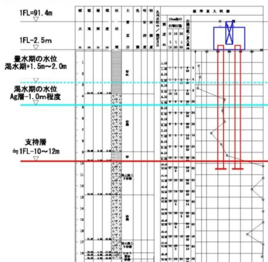
図 2-(1)-6 杭基礎
