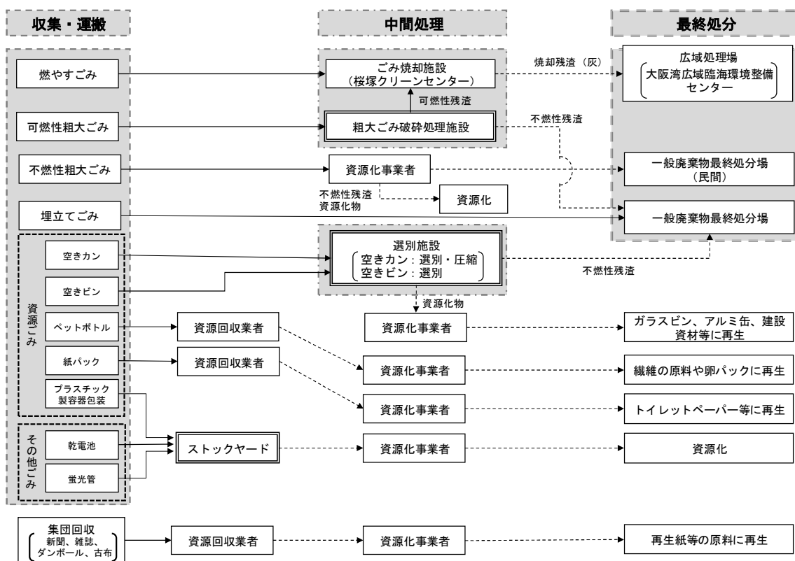
図 7-1 ごみ処理フロー
