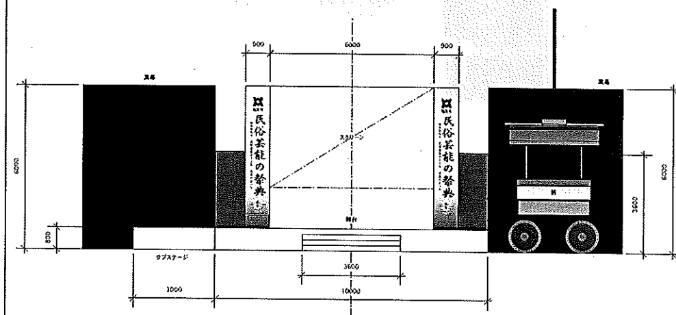
【立面図 ステージ】
